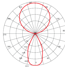
SDF-017-80W (4000K, 48deg)
